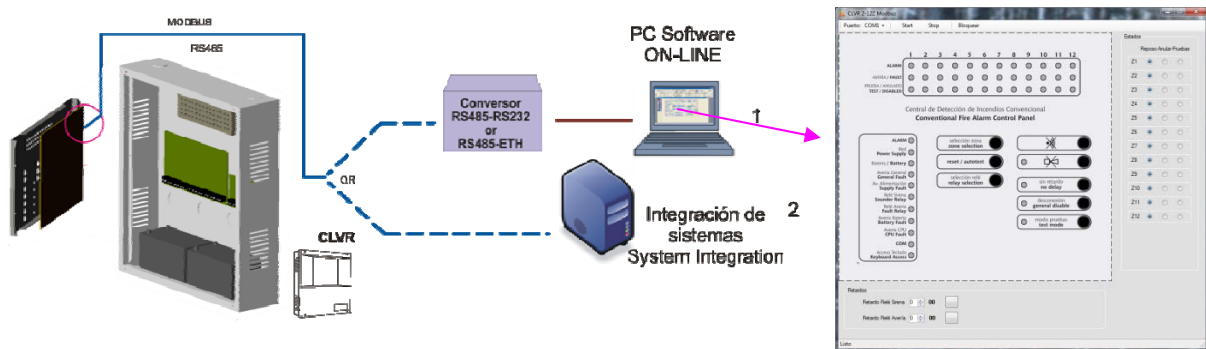
Figura 13 Comunicación MODBUS
