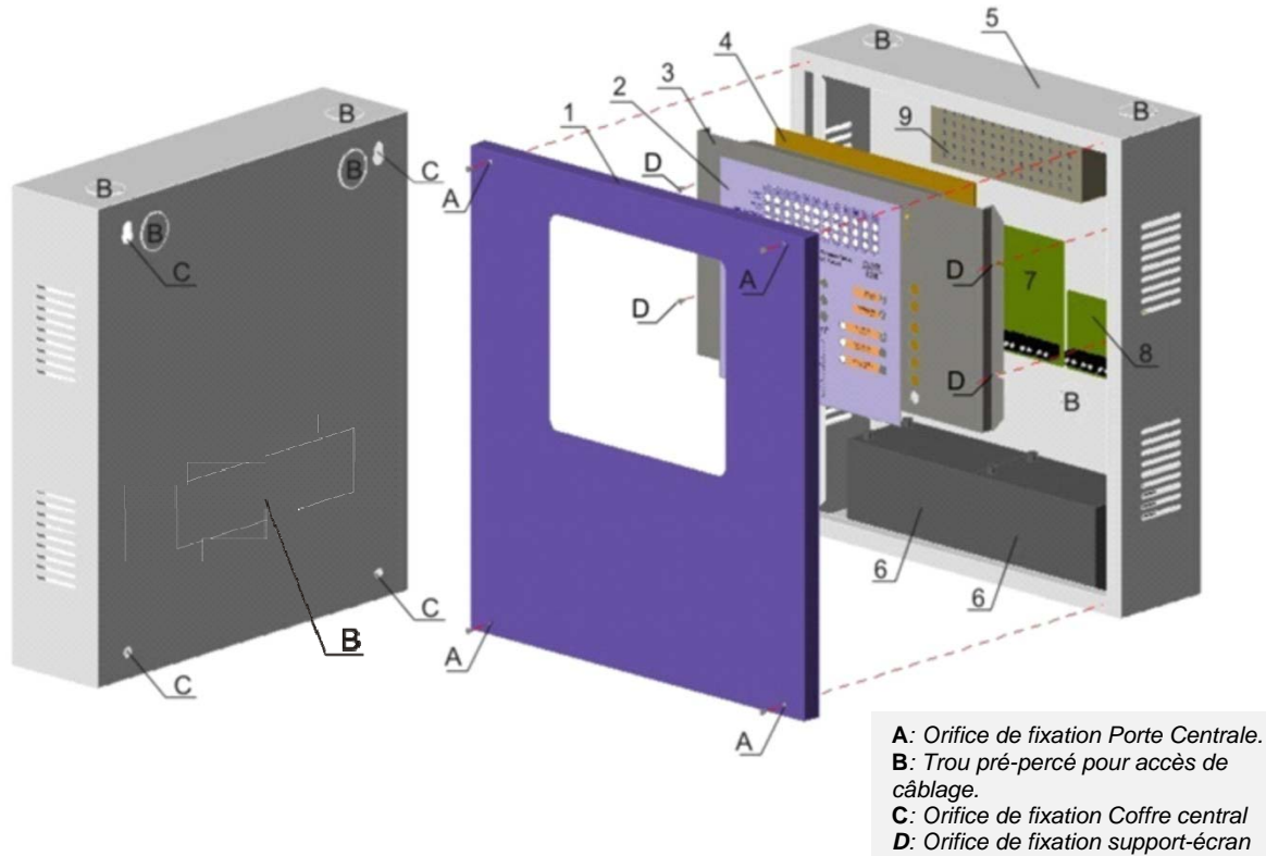
Figure 3 : Diagramme coffre et porte centrale.
