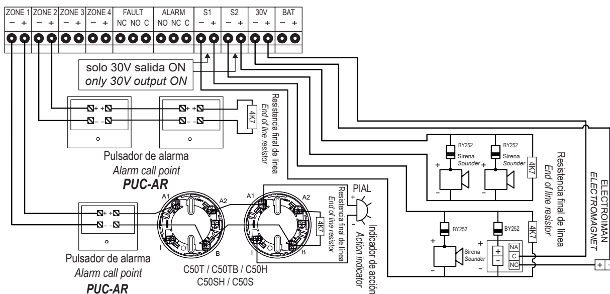
Esquema de conexionado para central IRON
