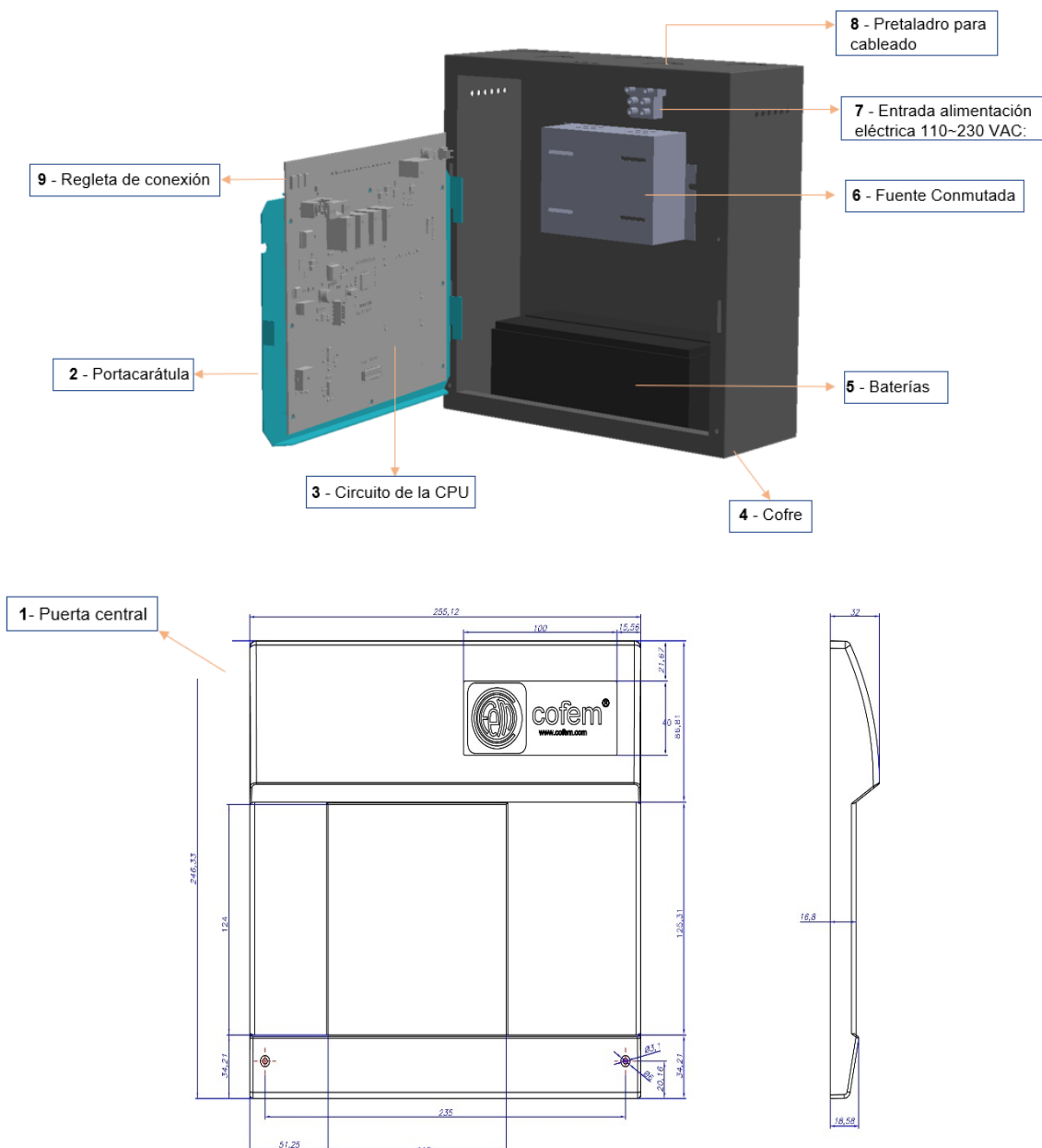
Figura 2: Diagrama cofre y puerta central
