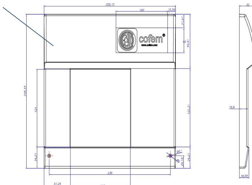
Figure 3 : Schéma coffre et porte de la centrale
